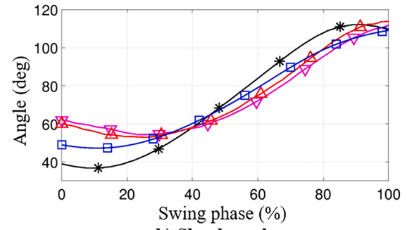
b) Shank angle
